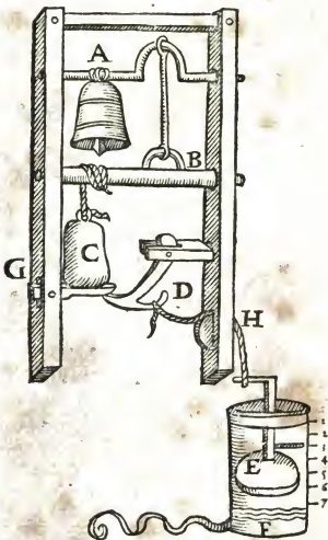
A Tintinnabulum. B Axis, cui alligatur funis, à quo pondus aliquod pendeat. C Pondus. G Lignum in quo pondus quic-
